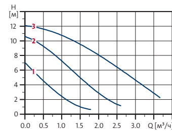
UPS 25-120 180
