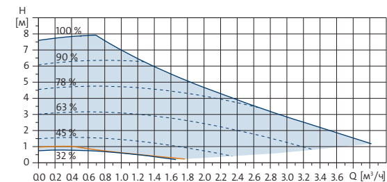
ALPHA3 XX-80
